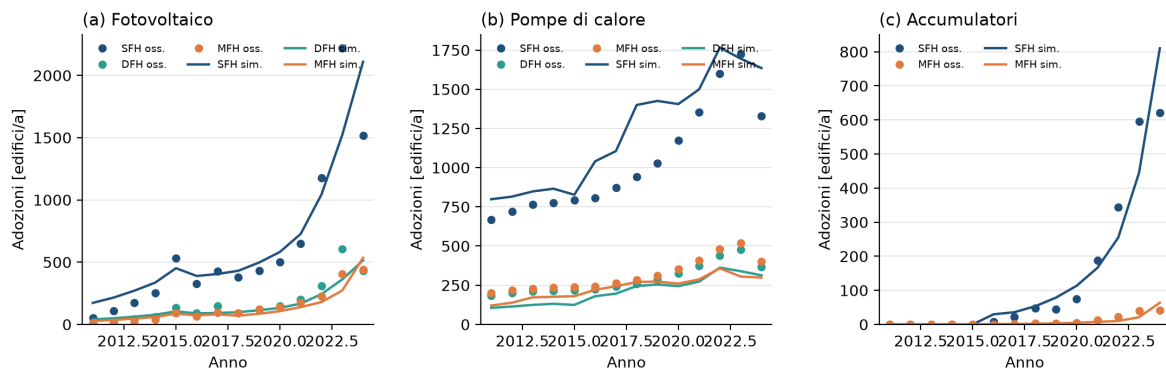
Figura 5.1: Flussi annuali di adozione: osservato (punti) e simulato (linee), 2011–2024. (a) Fotovoltaico per tipologia edilizia. (b) Pompe di calore per tipologia edilizia. (c) Accumulatori residenziali per tipologia.
