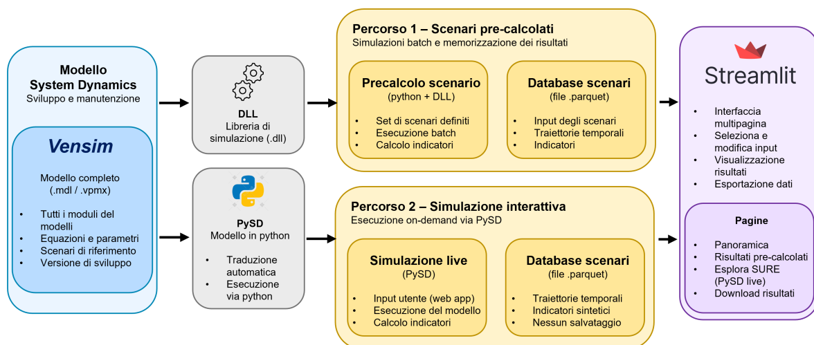
Figura 6.1: Architettura software del modello SURE-Ticino e della web application. Il modello System Dynamics è sviluppato e mantenuto in Vensim e viene utilizzato attraverso due percorsi complementari. Nel primo, il backend Vensim/DLL genera offline scenari pre-calcolati, successivamente memorizzati in file Parquet e letti dall'interfaccia Streamlit. Nel secondo, quando una combinazione non è disponibile nello store o richiede l'esplorazione congiunta di più leve, il modello tradotto in PySD viene eseguito on-demand e i risultati sono restituiti alla web application.
