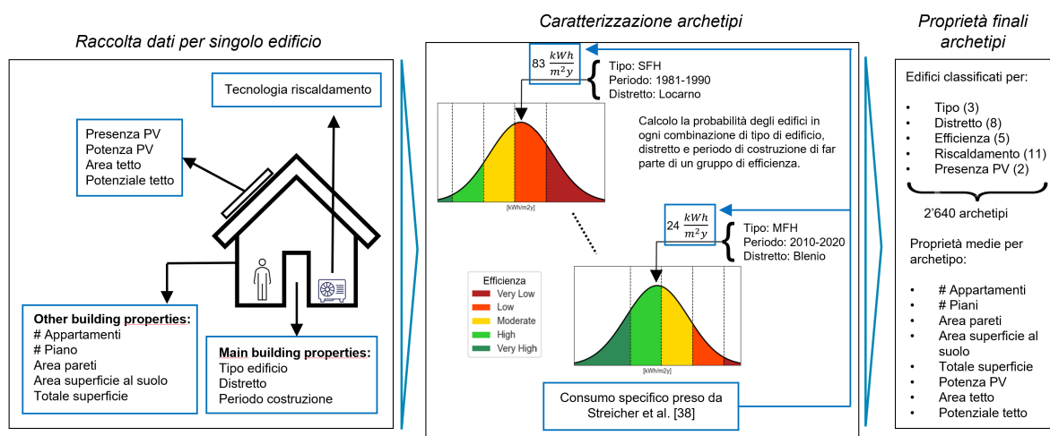
Figura 4.1: Procedura di costruzione degli archetipi residenziali utilizzati nel modello SURE-Ticino. I dati disponibili a livello di singolo edificio vengono integrati e utilizzati per classificare il patrimonio secondo tipologia edilizia, distretto, efficienza energetica, sistema di riscaldamento e presenza di PV. La procedura produce 2'640 archetipi, ai quali sono associate proprietà medie derivate dagli edifici appartenenti a ciascun gruppo.
