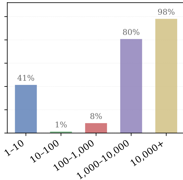
Top 5%
