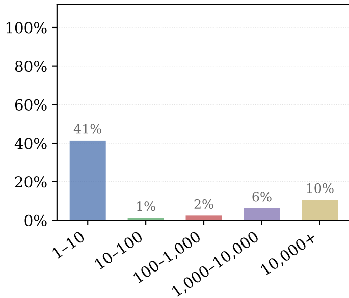
Top 1%
