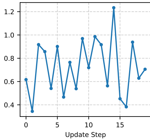
Gradient Norm
