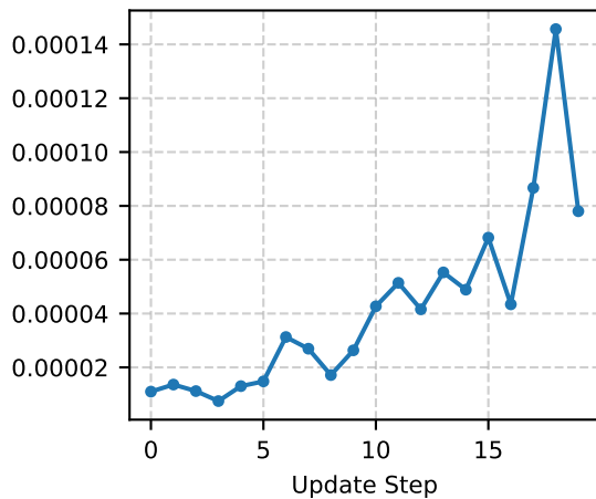
KL Divergence
