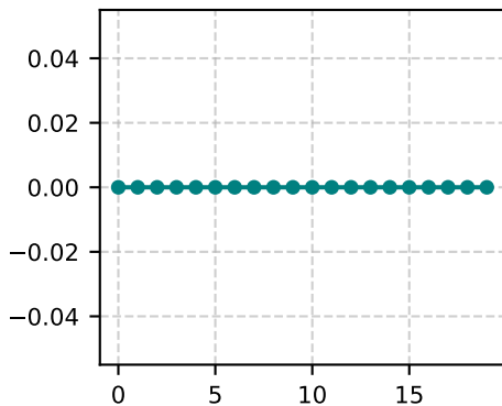
Clip Fraction
