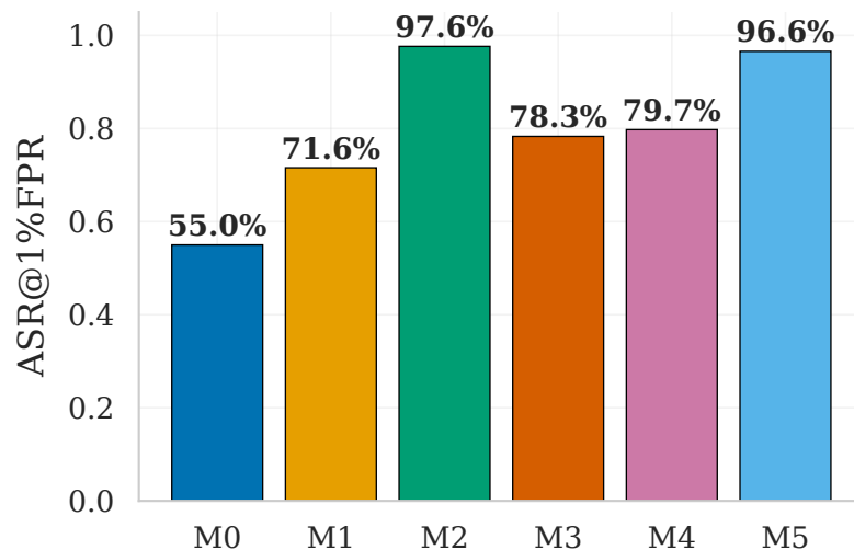
(d) Mean attack success
