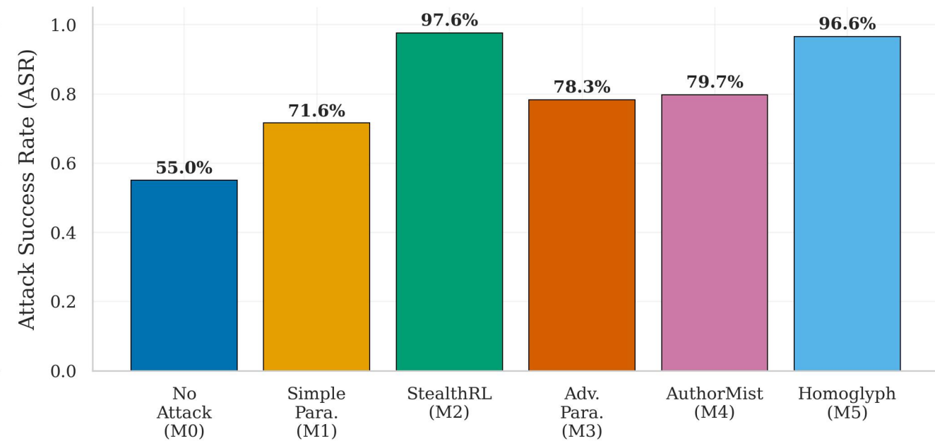
(d) Mean Attack Success Rate
