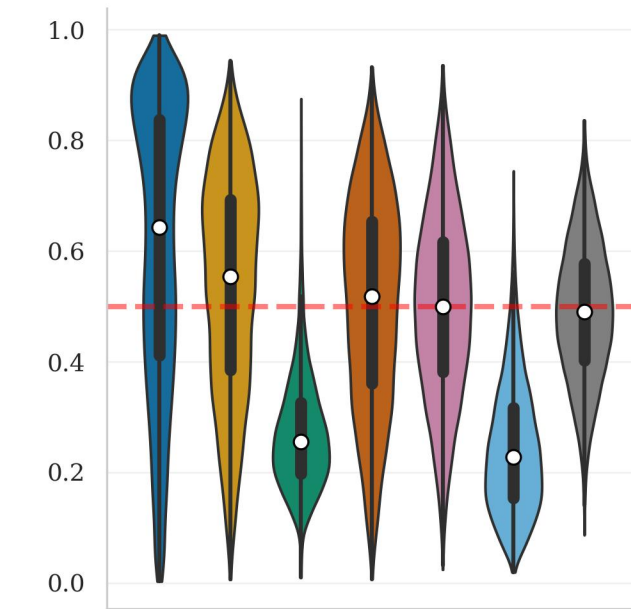
Fast Detectgpt
