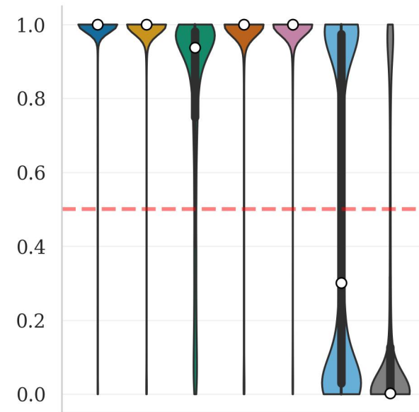
Mage
