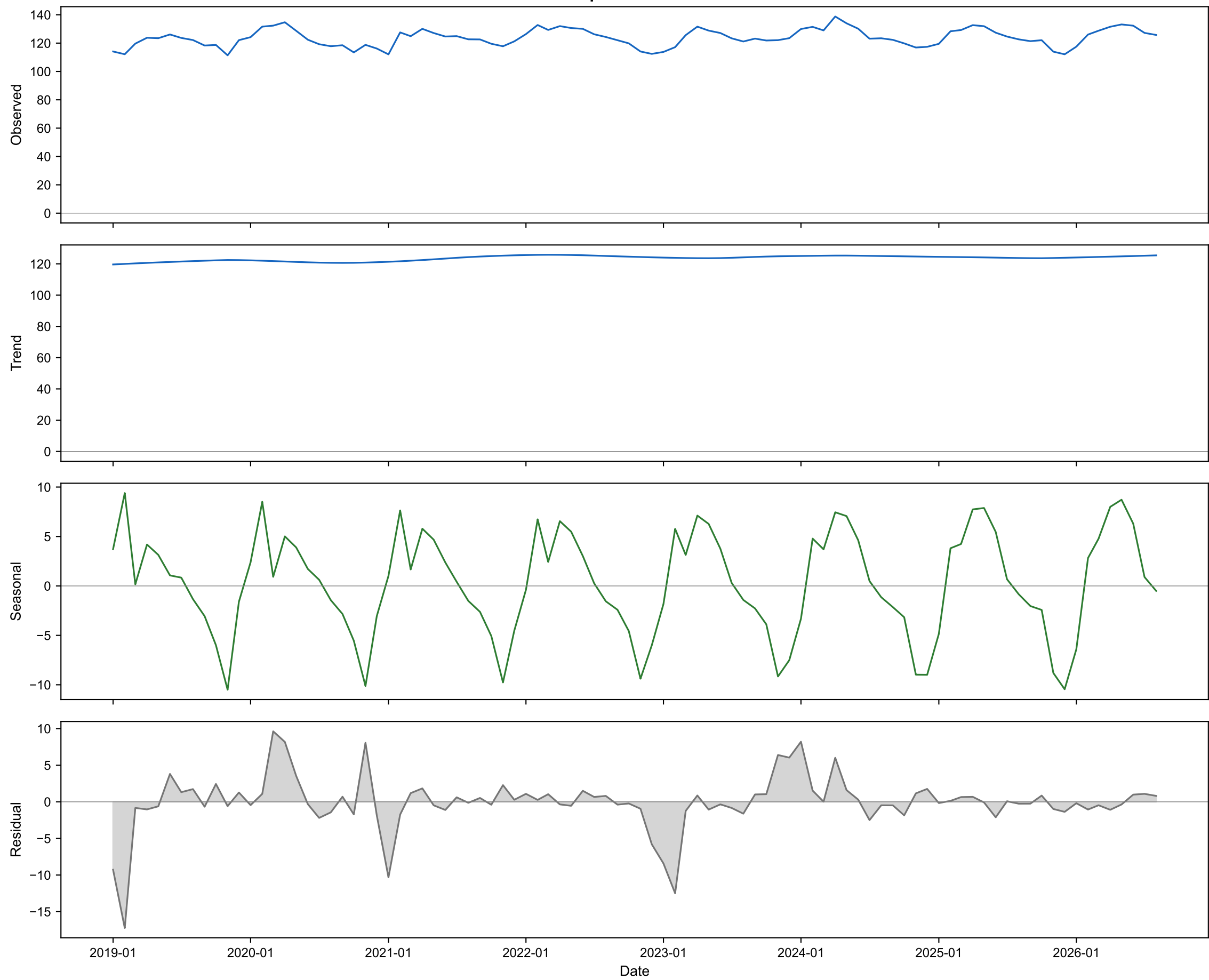
STL Decomposition: O3 — Siwalik
