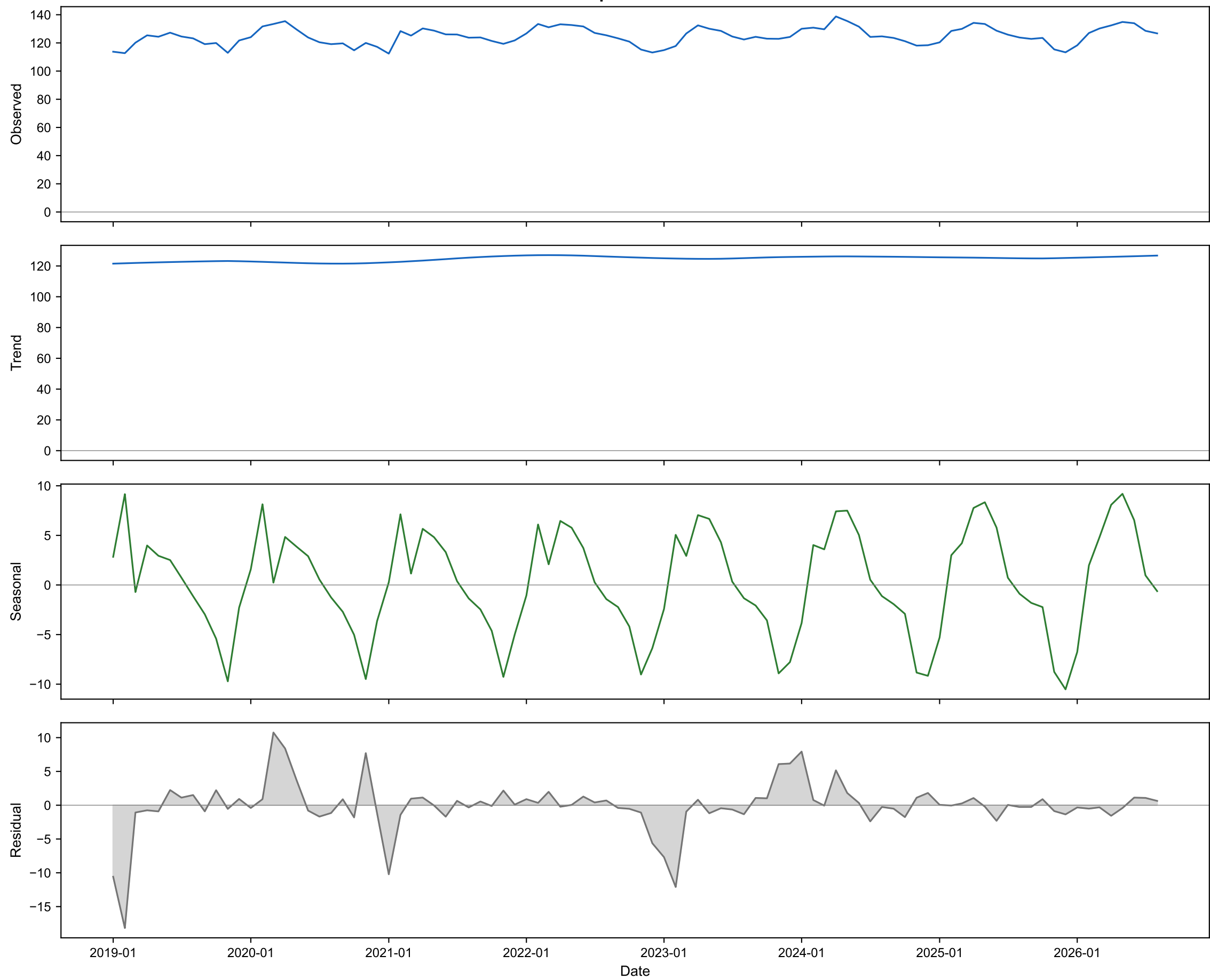
STL Decomposition: O3 — Terai
