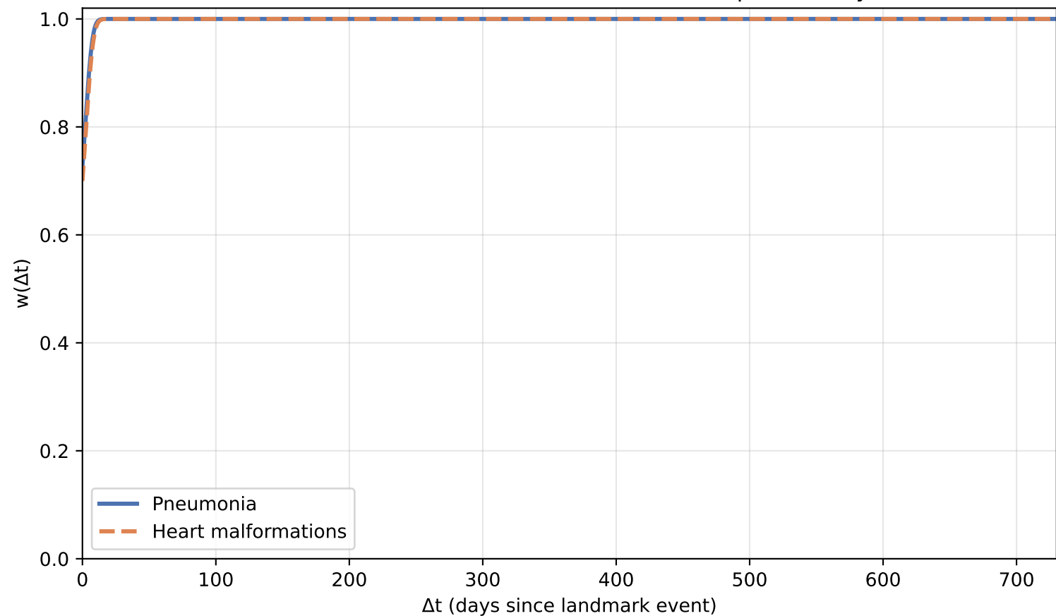
PIC fine-tuned · TALE-EHR · attention temporal decay
