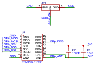
Lora
