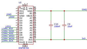
ESP32
