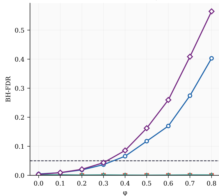
(d) BH False Discovery Rate
