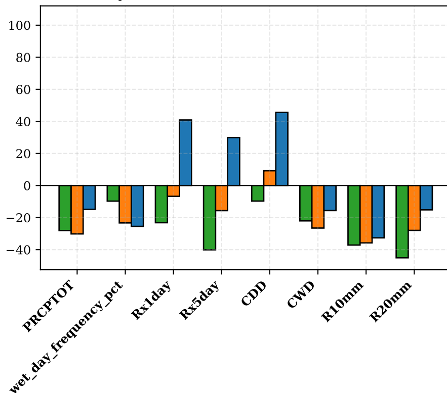
(c) Hot/Dry Season — El Niño
