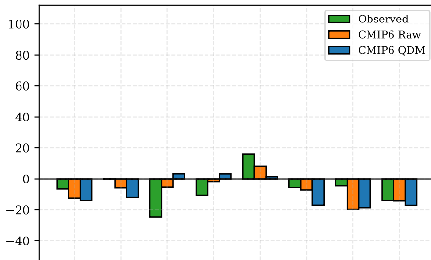
(a) Rainy Season — El Niño
