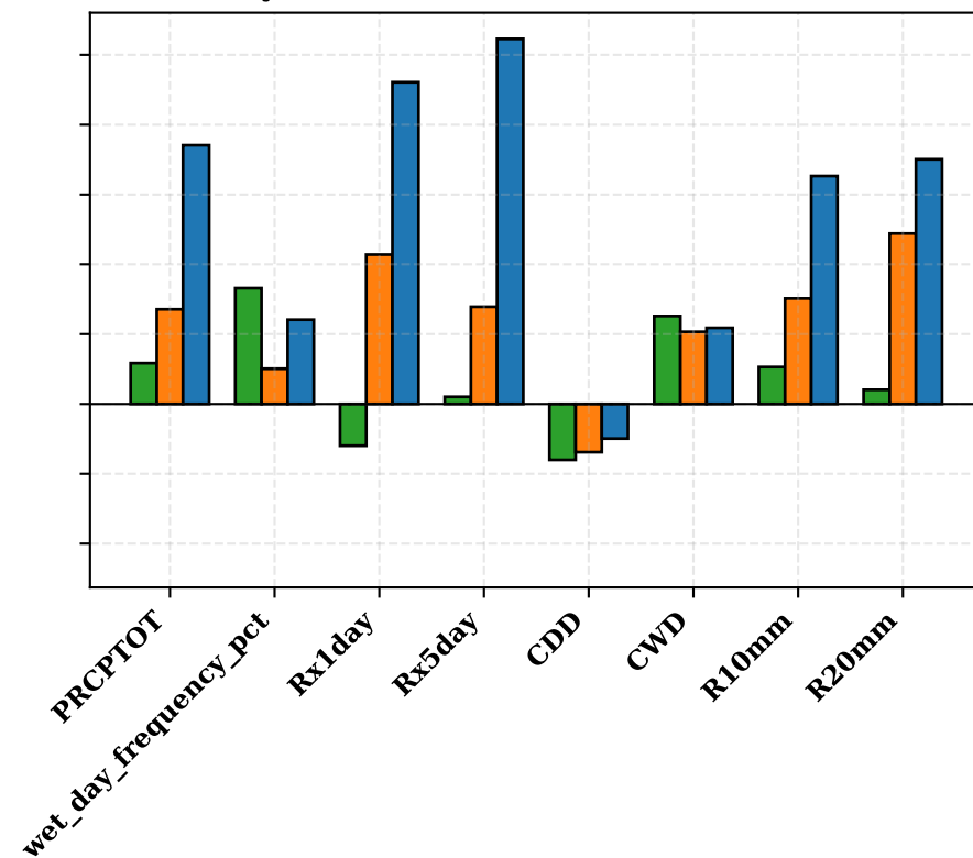
(d) Hot/Dry Season — La Niña
