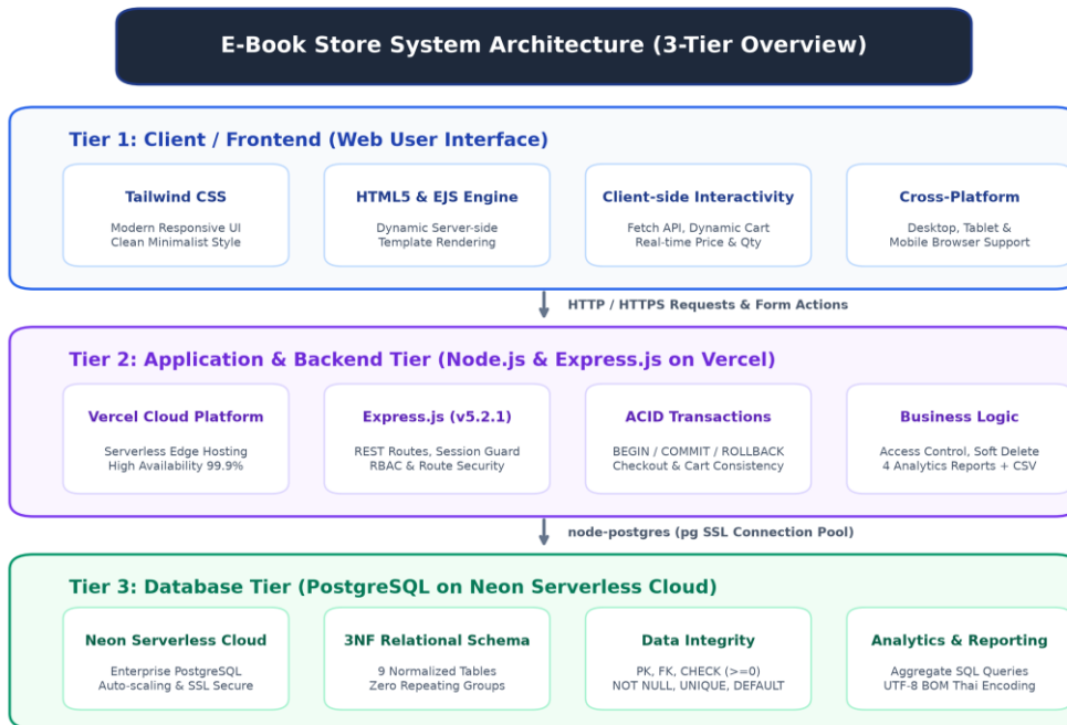
รูปที่ 1.1: ภาพรวมสถาปัตยกรรมระบบ 3 ระดับ (3-Tier System Architecture Overview)
