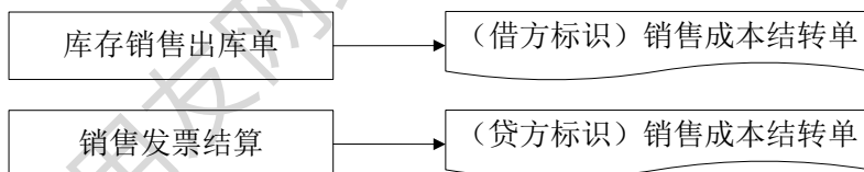
图 3.2-04 销售结算处理图
