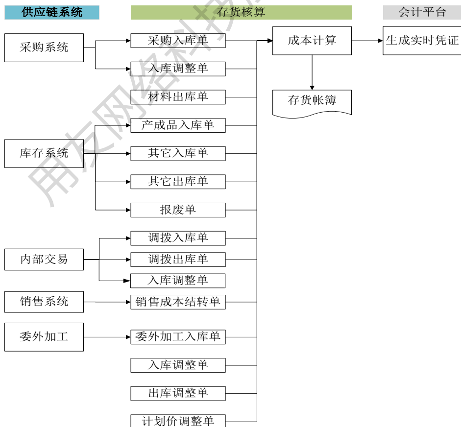
图 1.1-01 存货核算功能架构图
