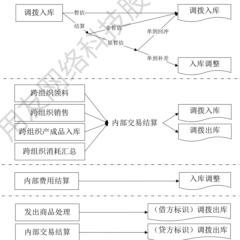
图 3.2-06 跨组织交易传存货核算示意图
