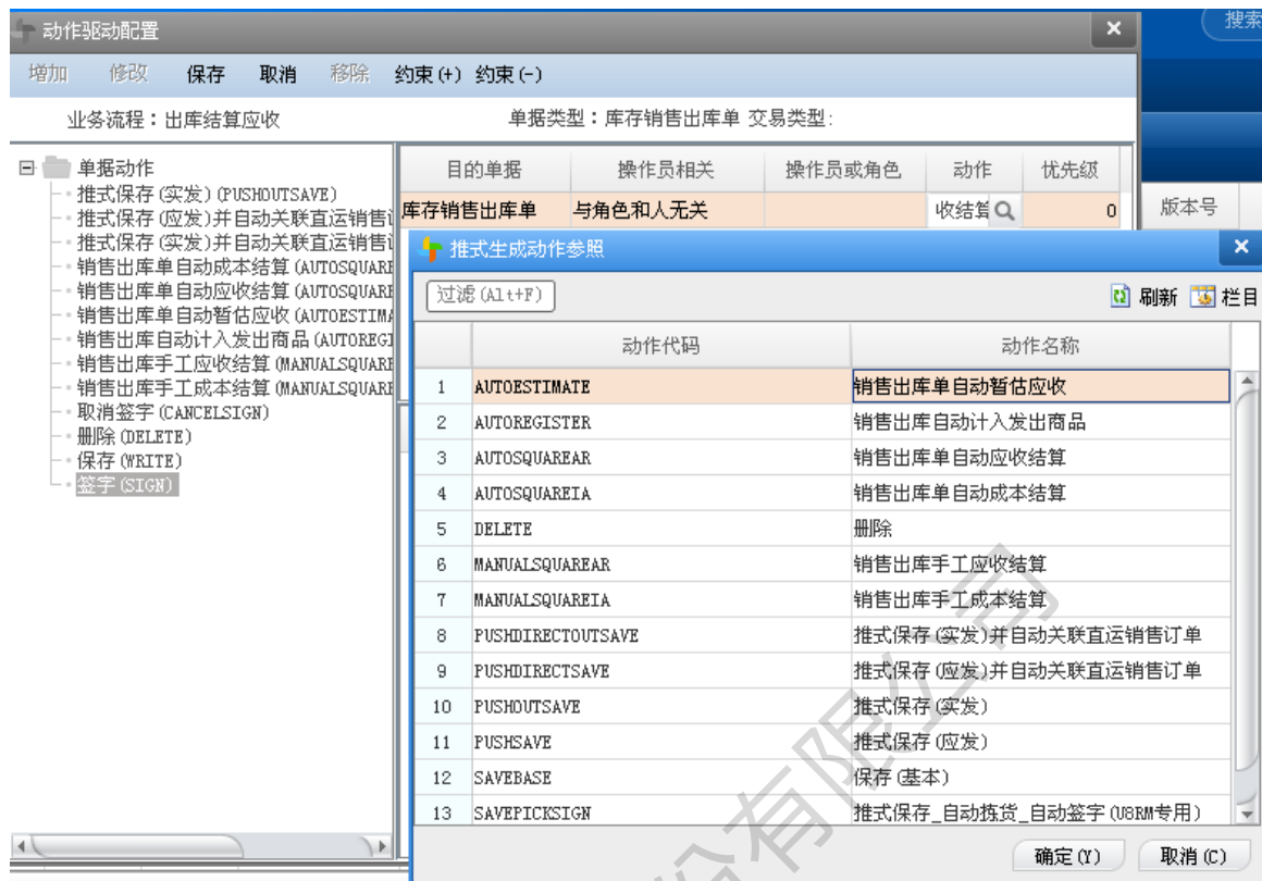
图 2.1.1-2 推式生成应收单的单据动作配置示例
