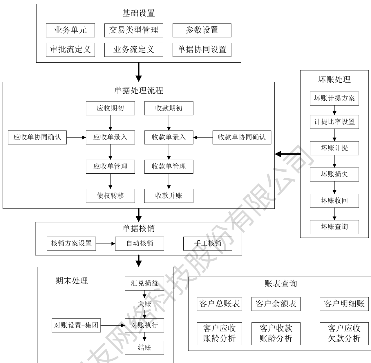
图 1.1-2 应收管理业务流程图
