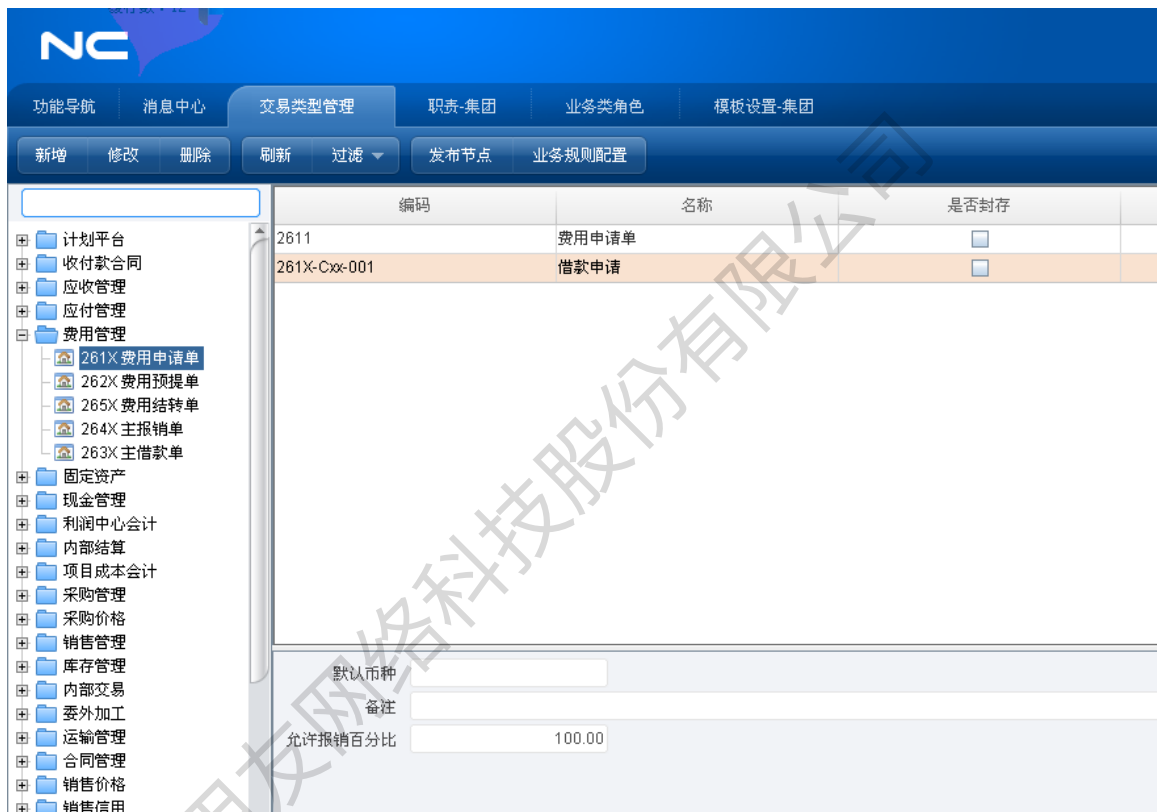
图 3.4-1 借款申请单
