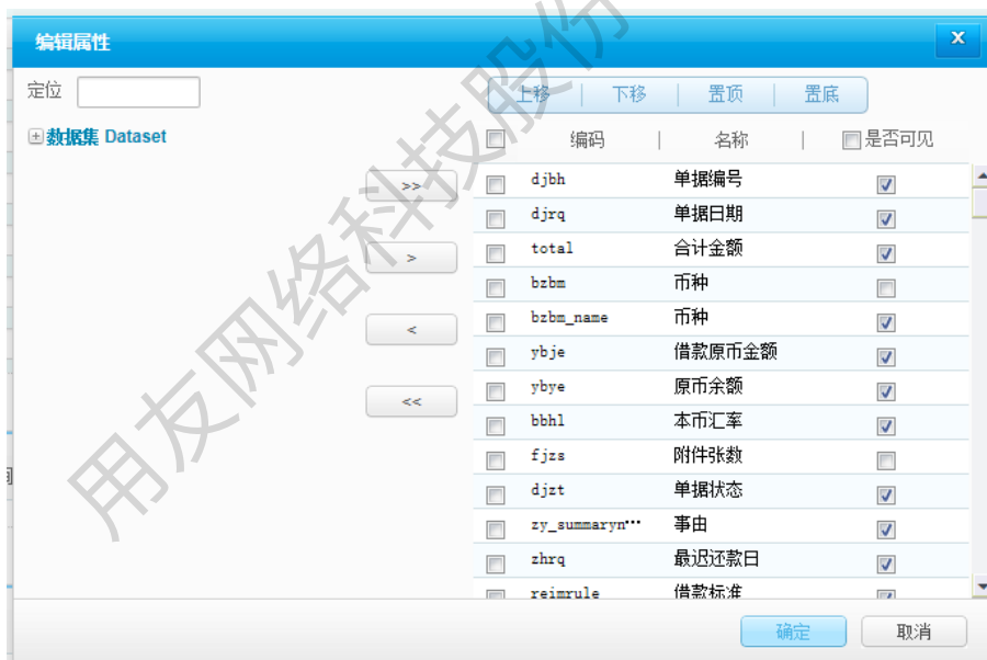
图 3.3-4 模板编辑
