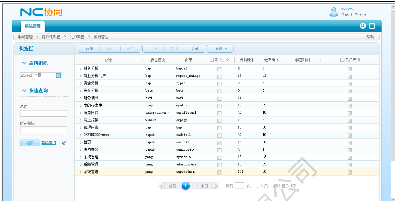
图 3.1-1 门户创建
