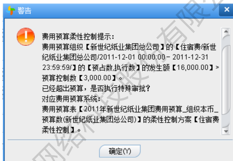
图 3.9-6 柔性控制
