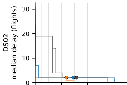
Residual PCA
