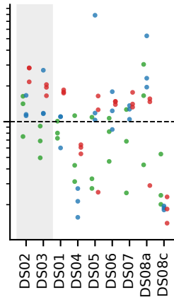
CVAE
