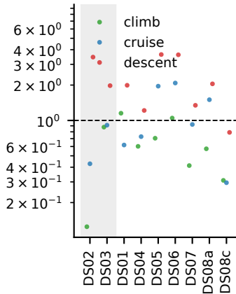
Residual PCA
