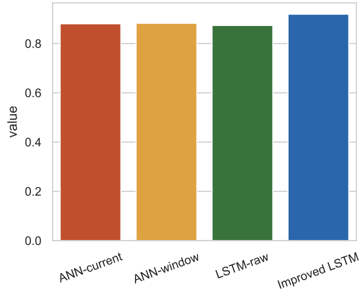
R2
