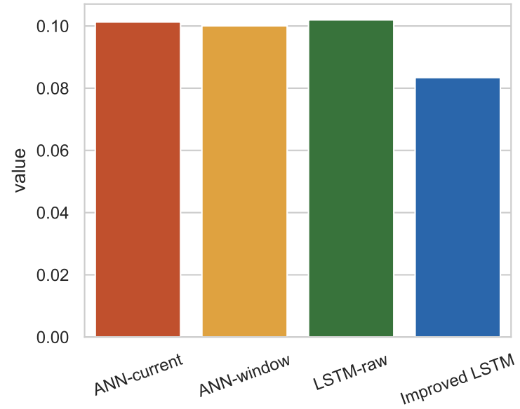
MAE
