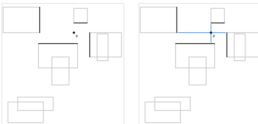
Figure 4: Zweiseitige Abbildung. Links ein Punkt p in der Szene mit acht Kästen, seine vier Cover schwarz, alle anderen Strecken grau. Rechts zusätzlich die beiden blauen Escape-Linien durch p , die kurz vor den Covern enden.
