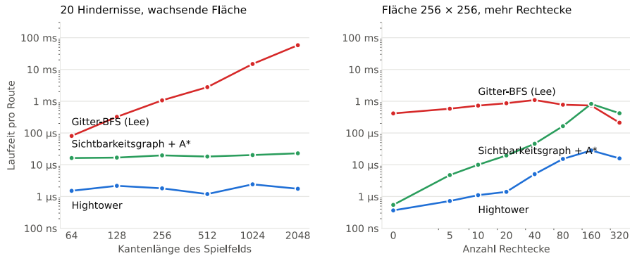
Figure 13: Zwei Liniendiagramme mit logarithmischer Zeitachse. Links wächst die Kantenlänge des Spielfelds von 64 auf 2048 bei 20 Hindernissen: die Breitensuche steigt von rund 80 Mikrosekunden auf 58 Millisekunden, der Sichtbarkeitsgraph bleibt bei 16 bis 23 Mikrosekunden, Hightower bei ein bis zwei Mikrosekunden. Rechts wächst die Zahl der Rechtecke von 0 auf 320 bei fester Fläche: die Breitensuche bleibt bei einer halben bis einer Millisekunde, der Sichtbarkeitsgraph steigt von unter einer Mikrosekunde auf über eine halbe Millisekunde, Hightower von 0,4 auf etwa 28 Mikrosekunden.
