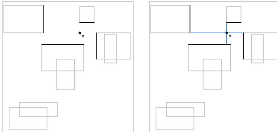
Figure 5: Zweiteilige Abbildung. Links ein Punkt p in der Szene mit acht Kästen, seine vier Cover schwarz, alle anderen Strecken grau. Rechts zusätzlich die beiden blauen Escape-Linien durch p , die kurz vor den Covern enden.
