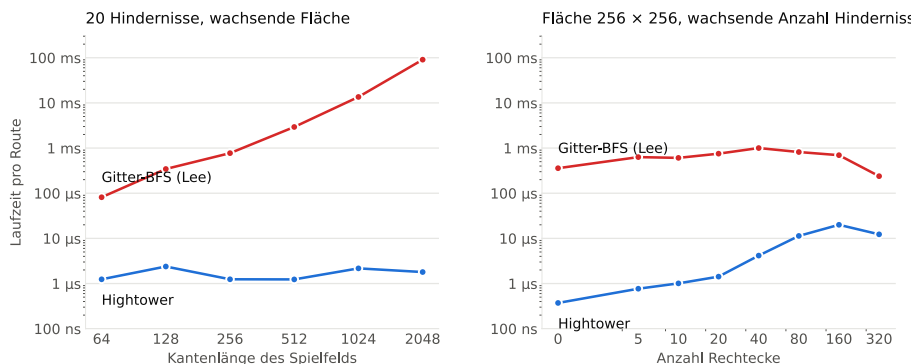
Figure 11: Zwei Liniendiagramme mit logarithmischer Zeitachse. Links wächst die Kantenlänge des Spielfelds von 64 auf 2048 bei 20 Hindernissen: die Breitensuche steigt von rund 80 Mikrosekunden auf 90 Millisekunden, Hightower bleibt bei ein bis zwei Mikrosekunden. Rechts wächst die Zahl der Rechtecke von 0 auf 320 bei fester Fläche: die Breitensuche bleibt bei einer halben bis einer Millisekunde, Hightower steigt von 0,4 auf etwa 20 Mikrosekunden.
