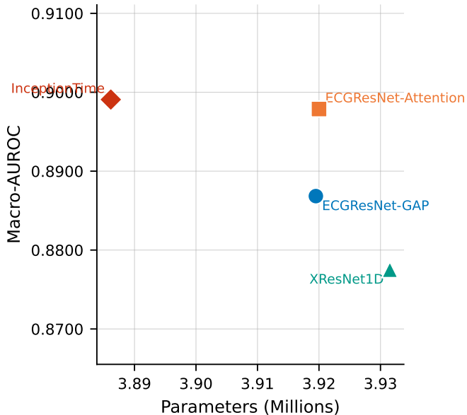
(A) Macro-AUROC vs. Parameters
