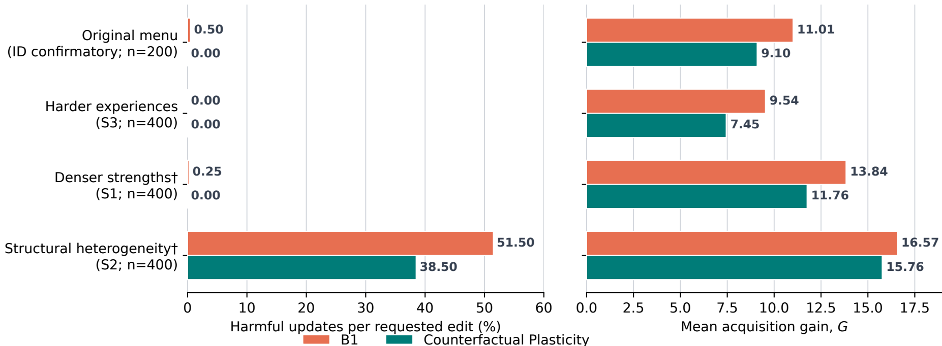
Harmful-update rate
