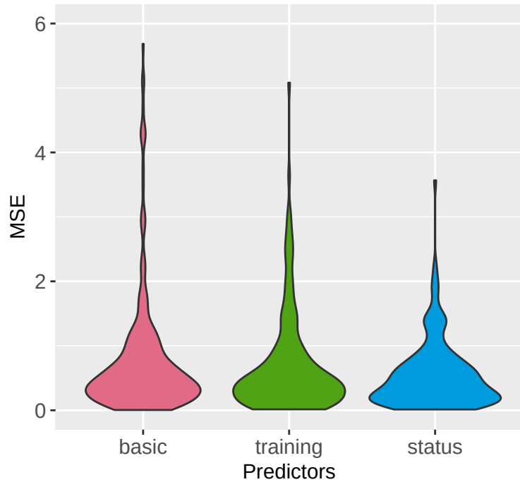
Lasso Regression
