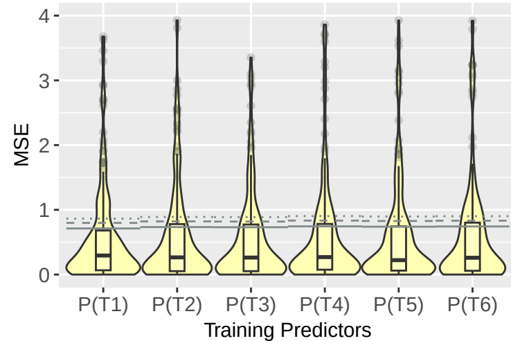
O(T6)
