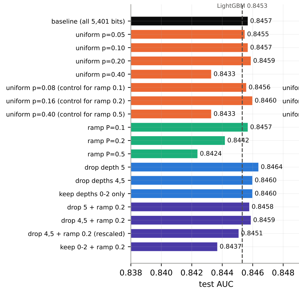
Test AUC
