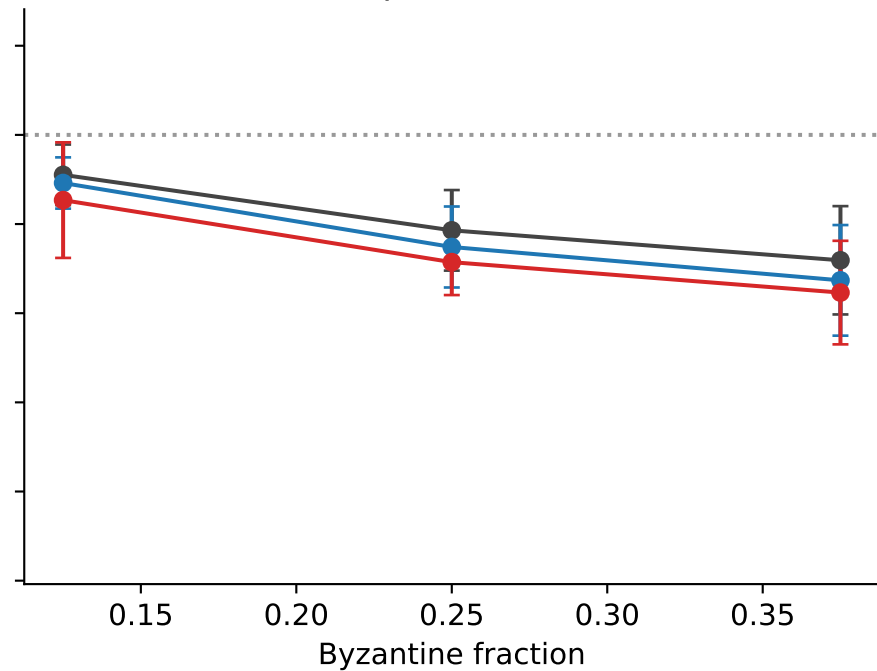
adaptive (ALIE)
