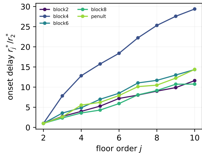
ViT-8 / C10
