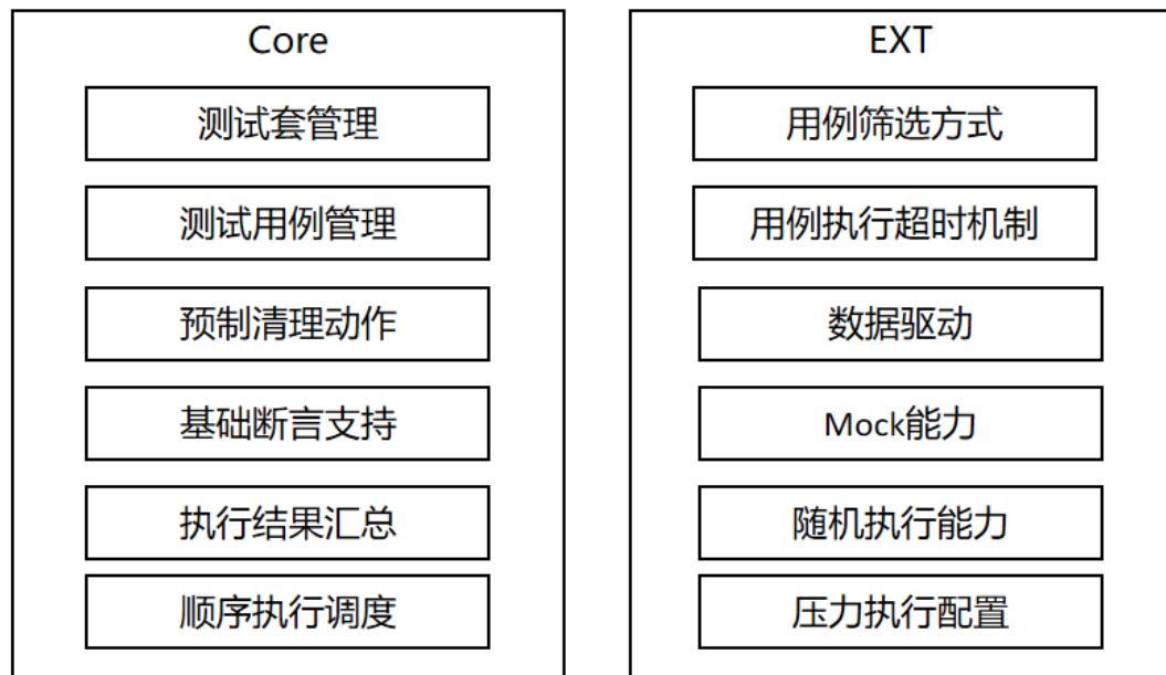
单元测试框架
