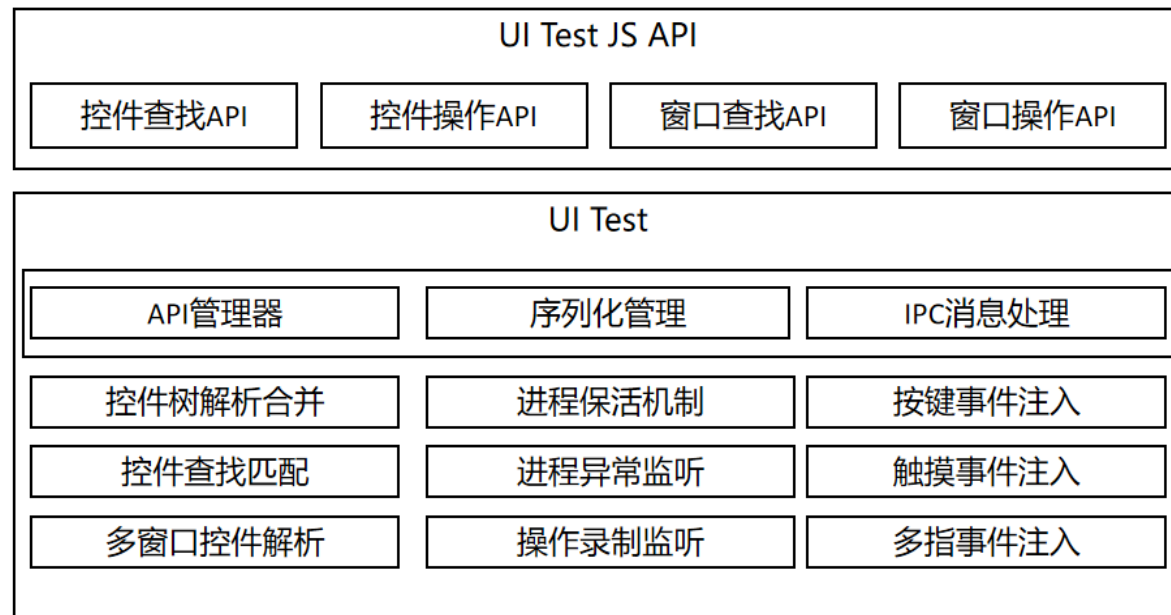
UI测试框架
