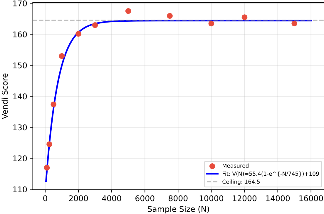
(d) Vendi Scaling Law ( R^2=0.996 )
