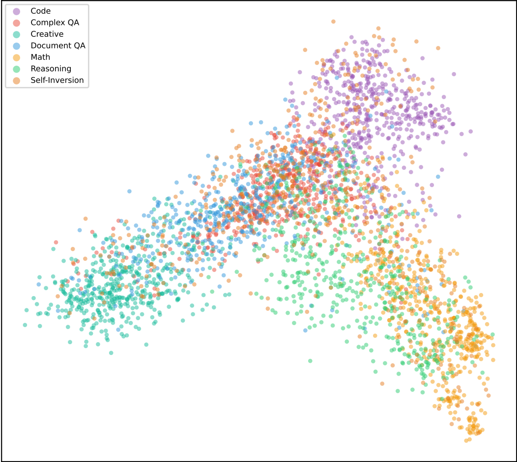
(a) PCA (var=9.2%)
