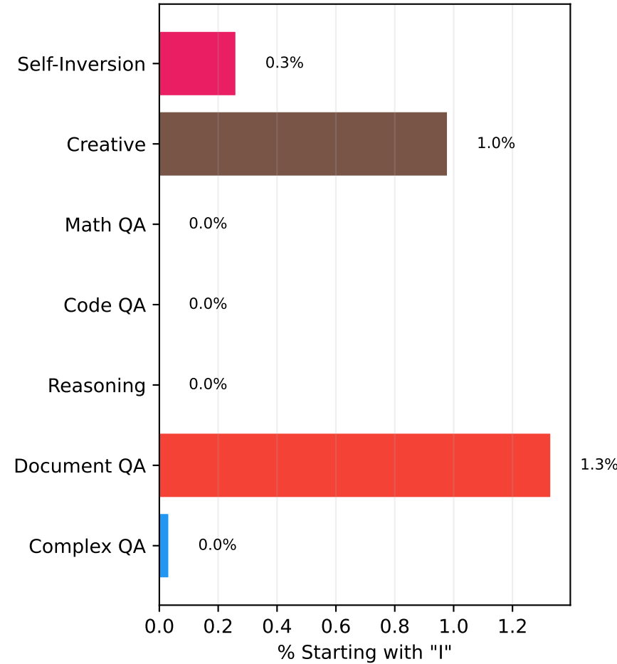
(d) First-Person Start Rate
