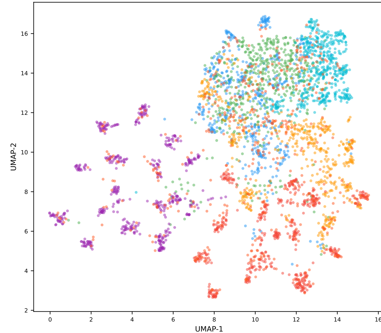
UMAP (n=50, d=0.5, cosine)
