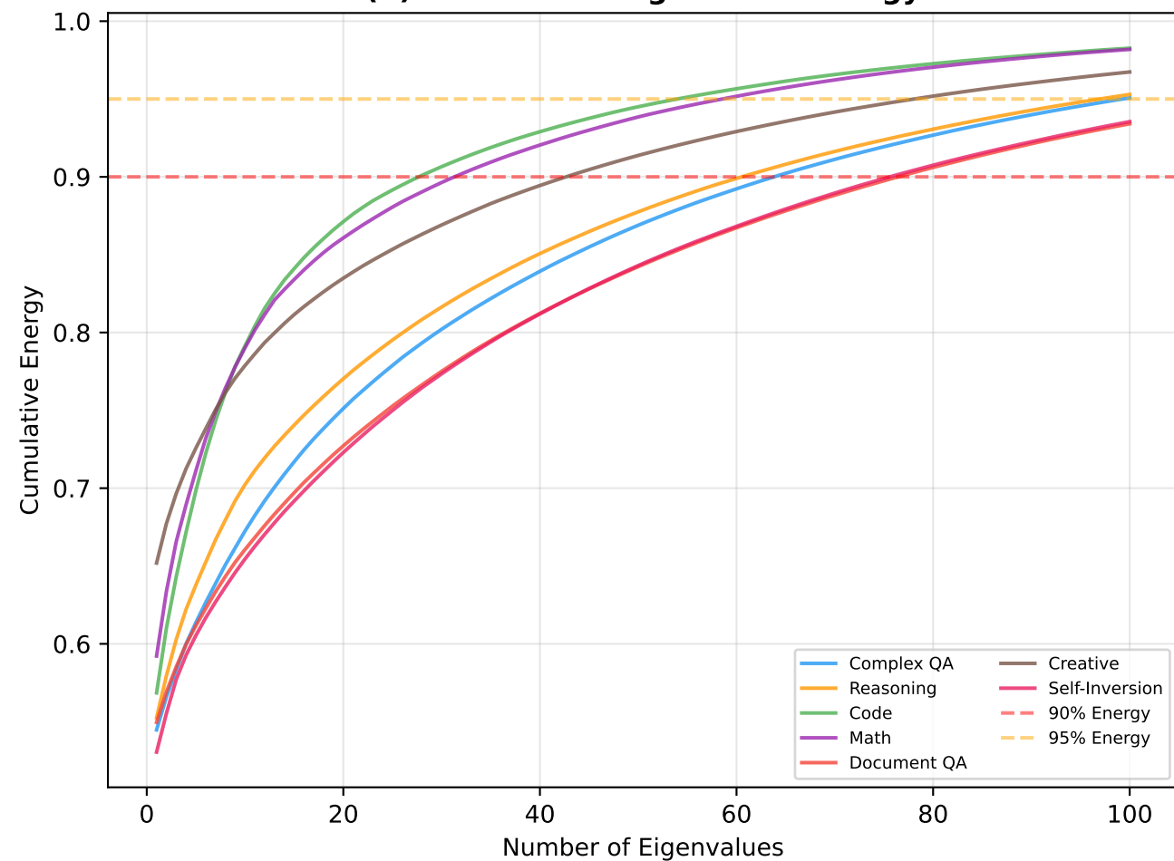
(d) Full Dataset Spectrum (Vendi=20.3)
