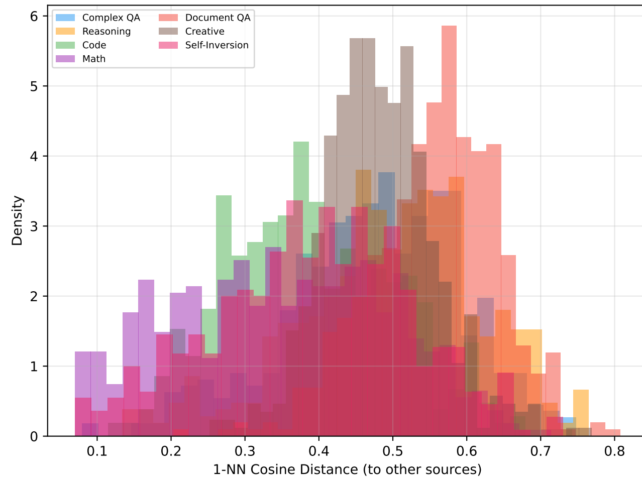
(d) Per-Sample Isolation Distribution
