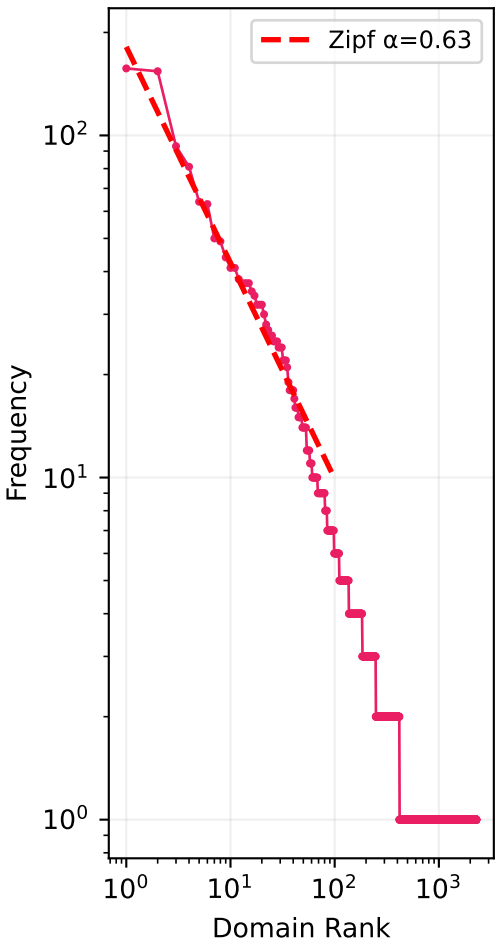
(d) Domain Zipf (2,288 unique)
