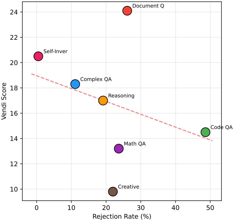
(d) Rejection vs Diversity (r=-0.315)
