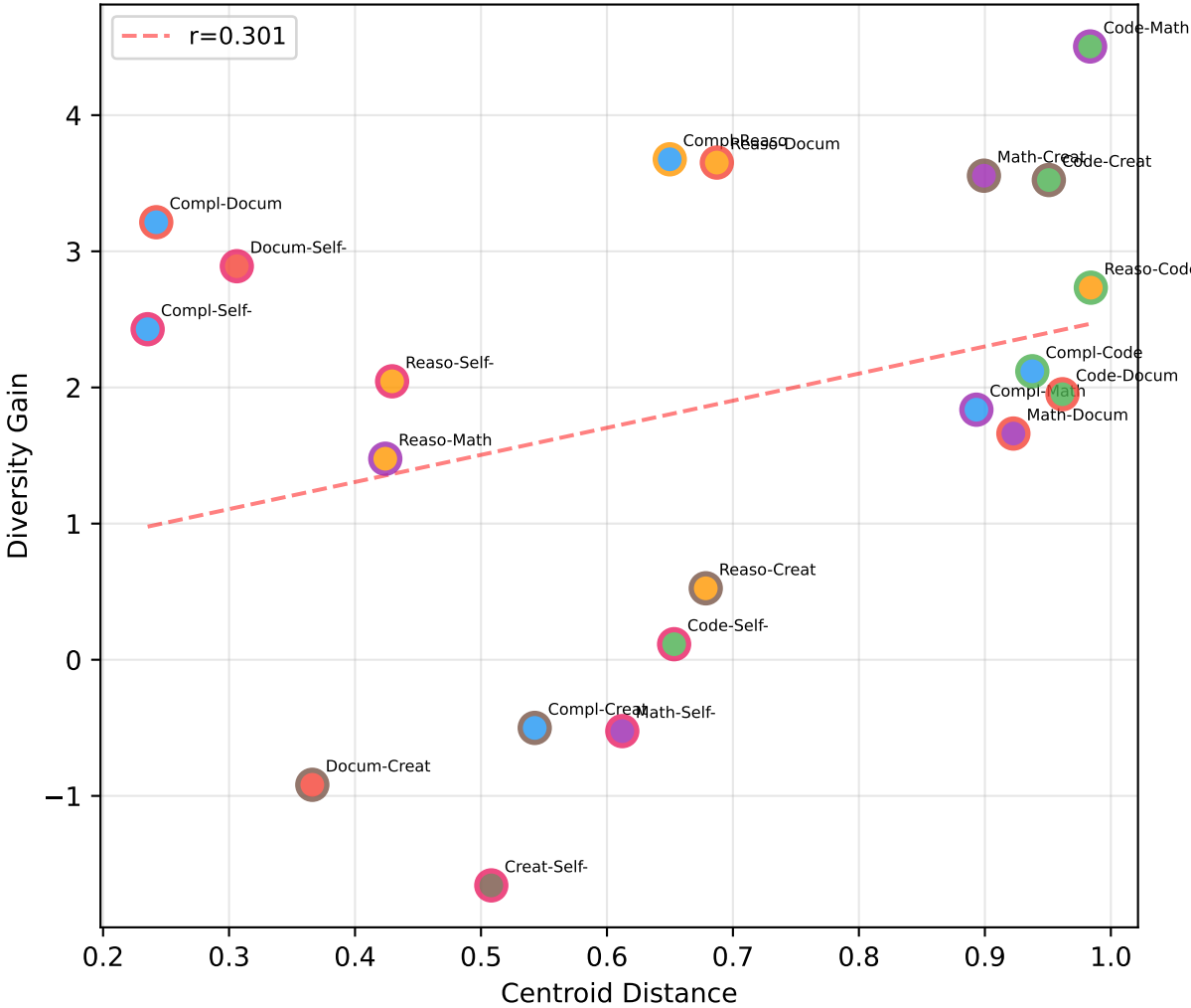
(d) Distance vs Synergy
