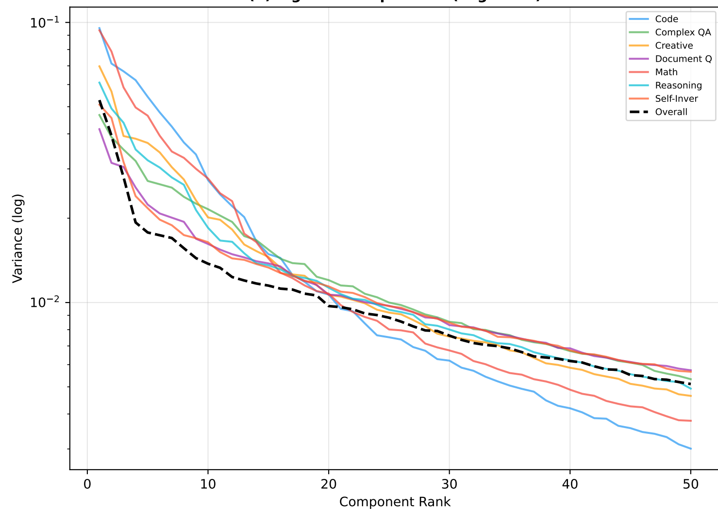
(d) Eigenvalue Spectrum (Log Scale)
