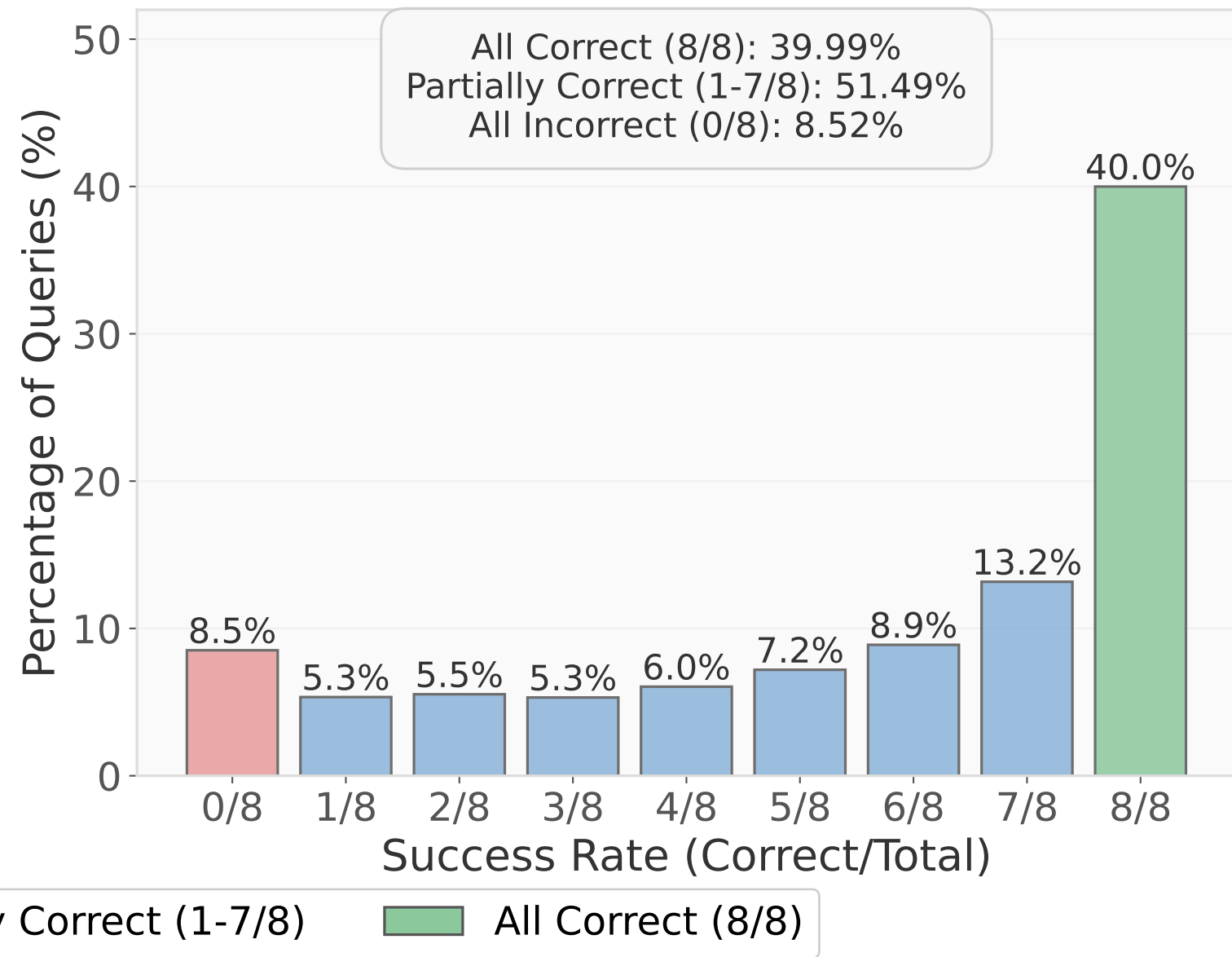
Qwen3.5-397B-A17B
