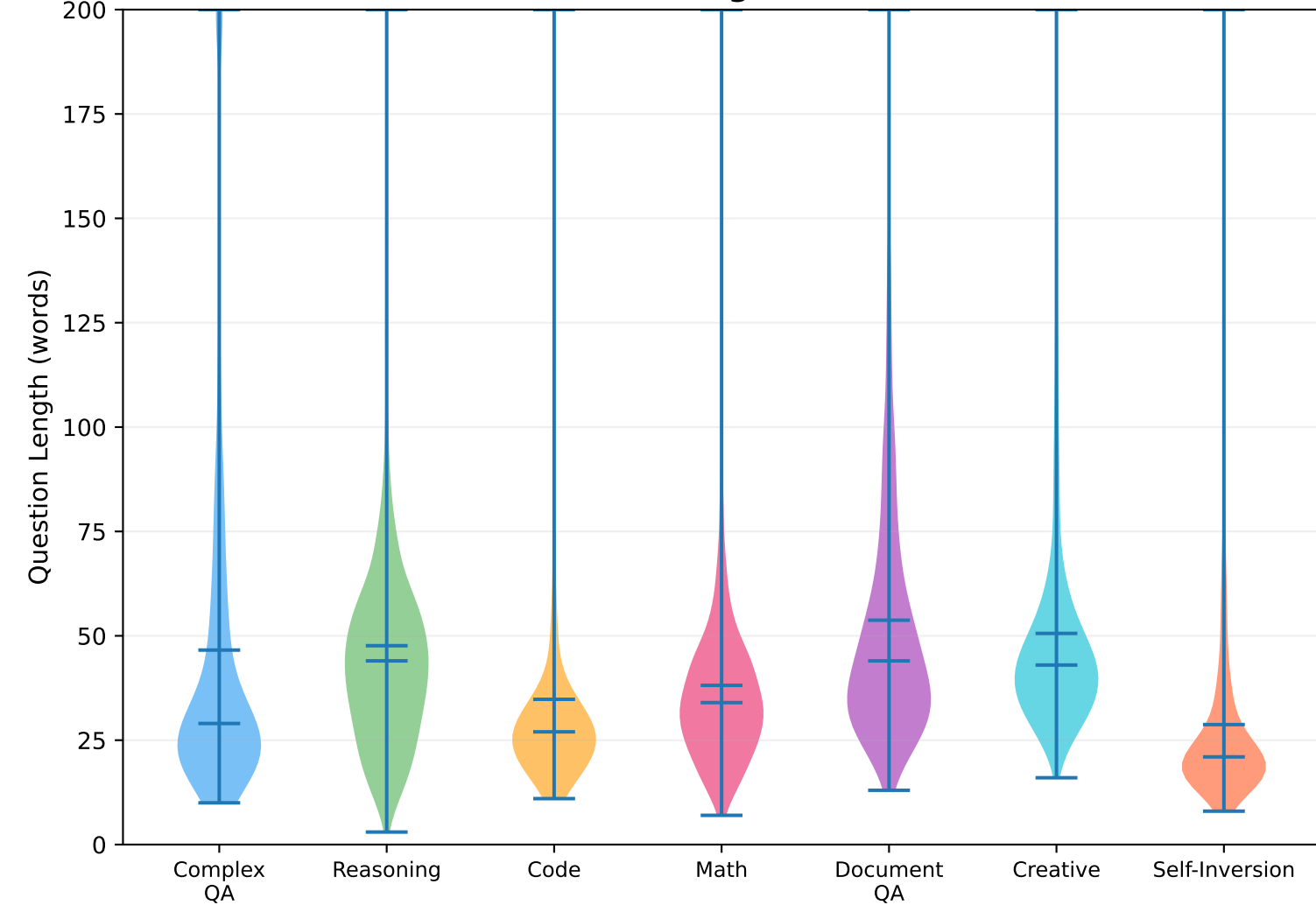
(d) Question Length Distribution
