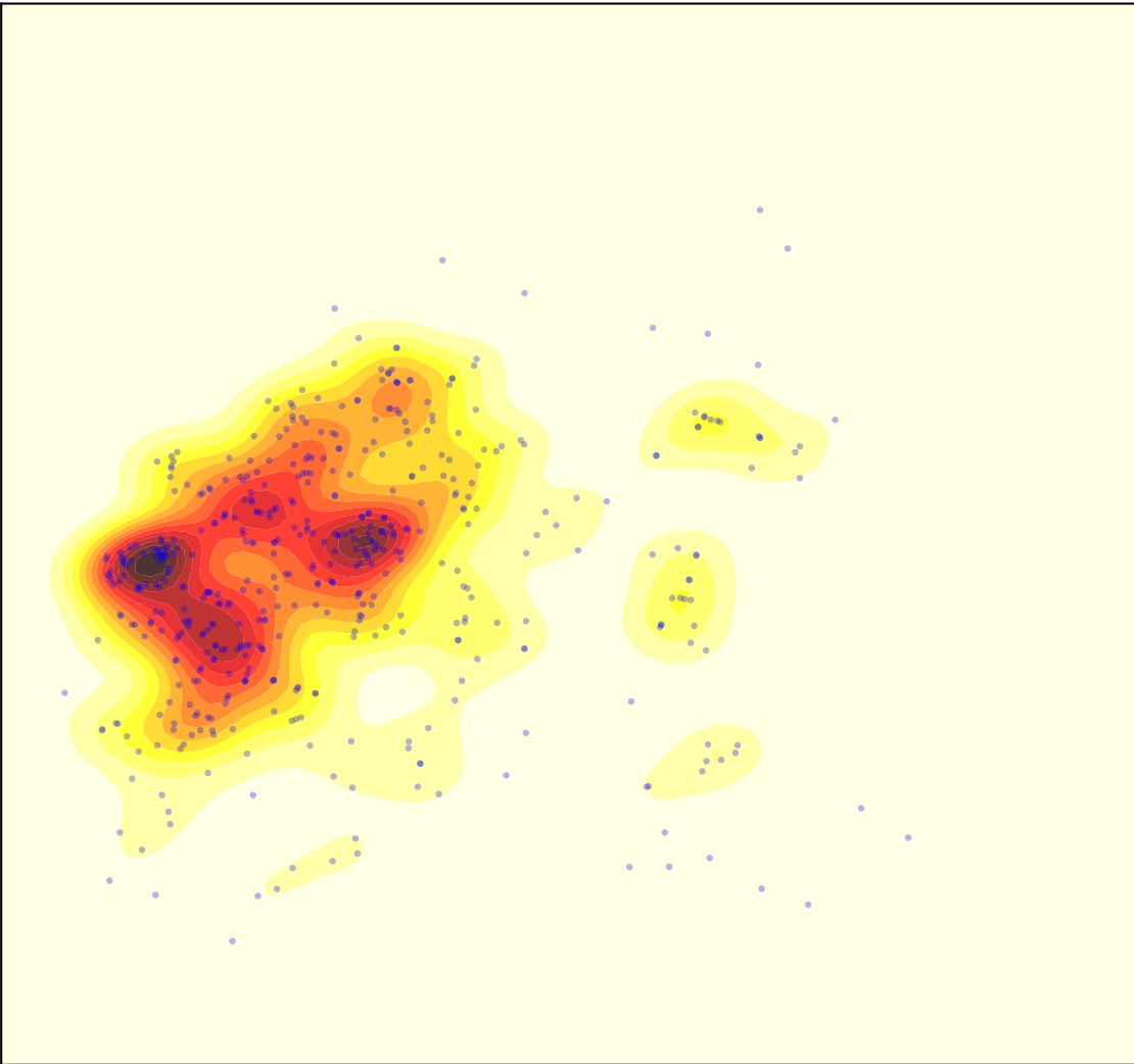
Document QA
