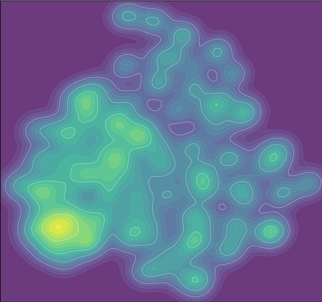
Document QA
