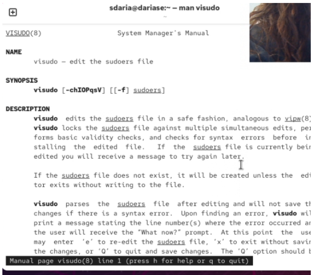
Рисунок 3.9: Справочное описание команды visudo
