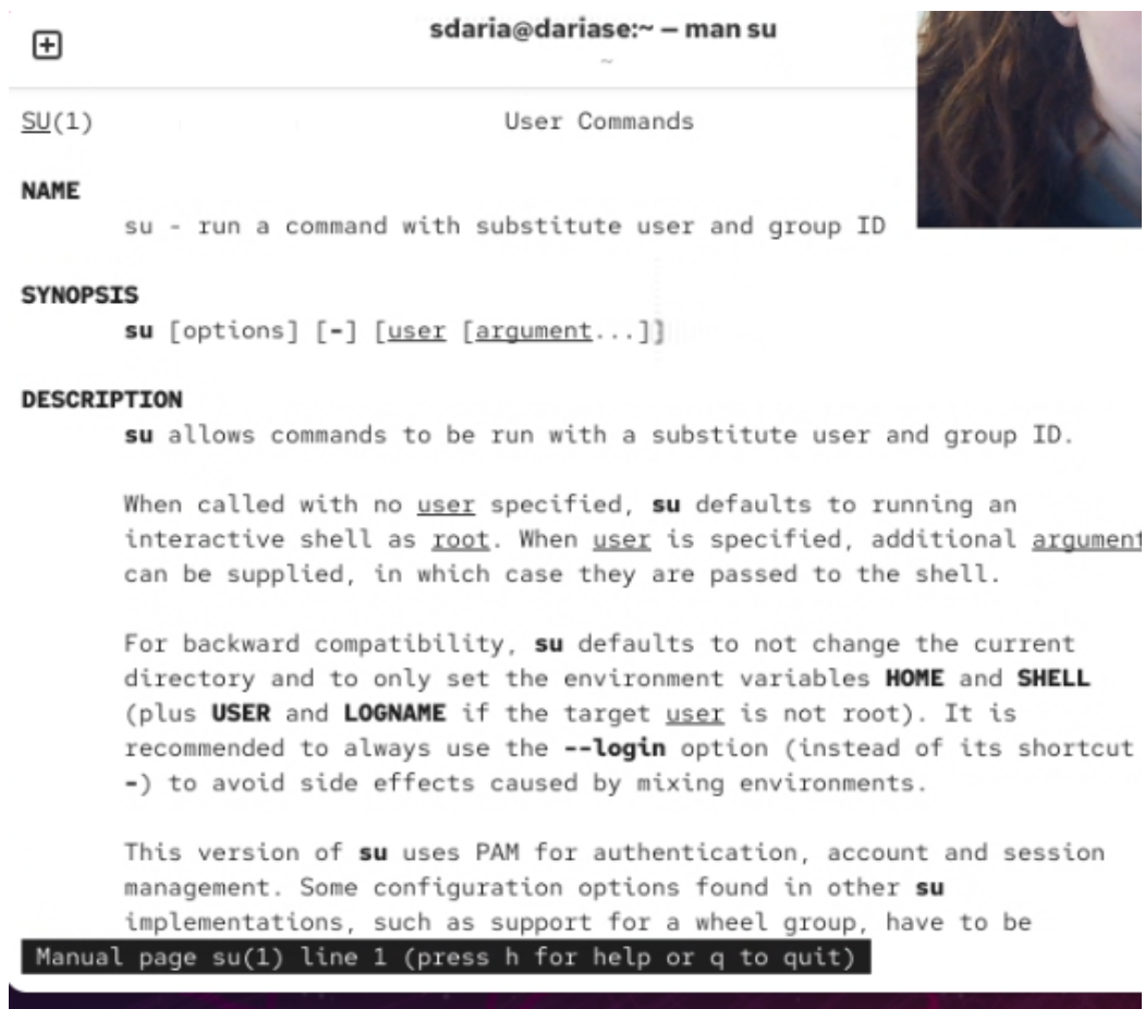
Рисунок 3.5: Справочное описание команды su
