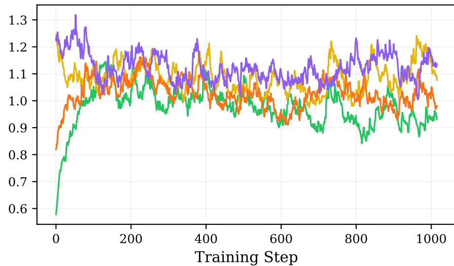
Gradient Norm
