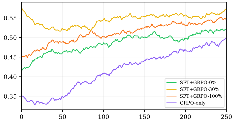
KL Loss
