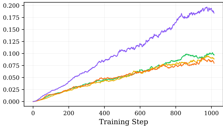
KL Loss
