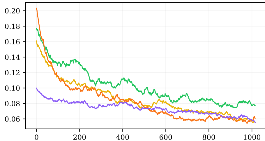
Gradient Norm
