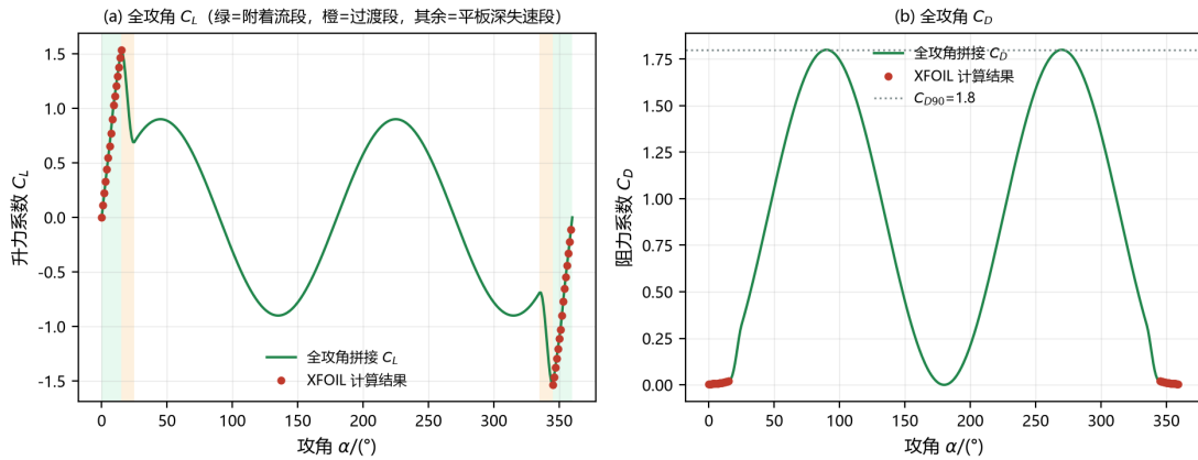
图 7 全攻角极线的三段式拼接结果
