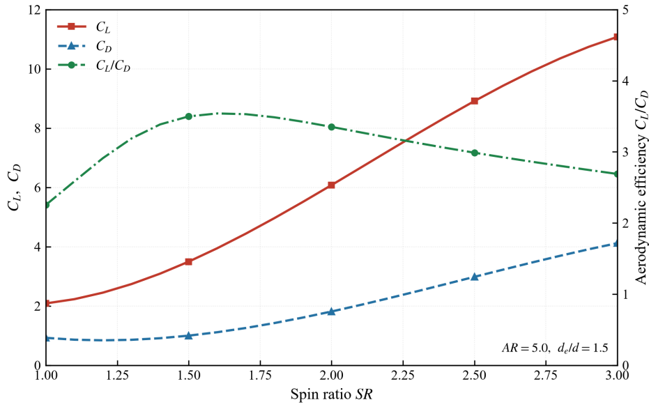
图 8 转筒帆升阻力系数与气动效率随转筒比的变化 ( AR = 5.0 , d_e/d = 1.5 )
