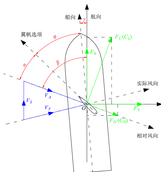
图 5 风翼受力简图 ( \beta 、 \alpha 、 \varphi 为本文所用角度体系)
