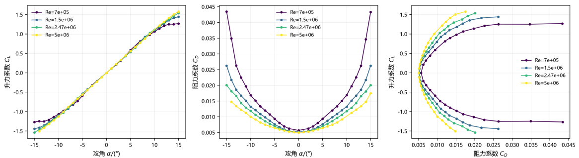
图 6 翼帆翼型极线的 XFOIL 计算结果
