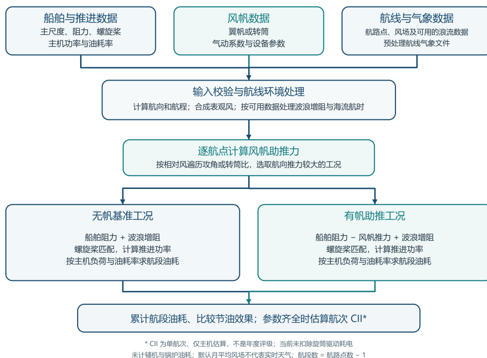
图 1 风帆助推船舶航次能耗计算流程
