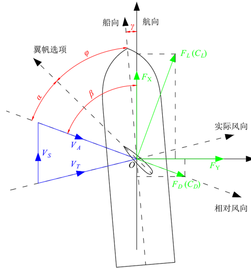
图 2 风翼受力简图 ( \beta 、 \alpha 、 \varphi 为本文所用角度体系)
