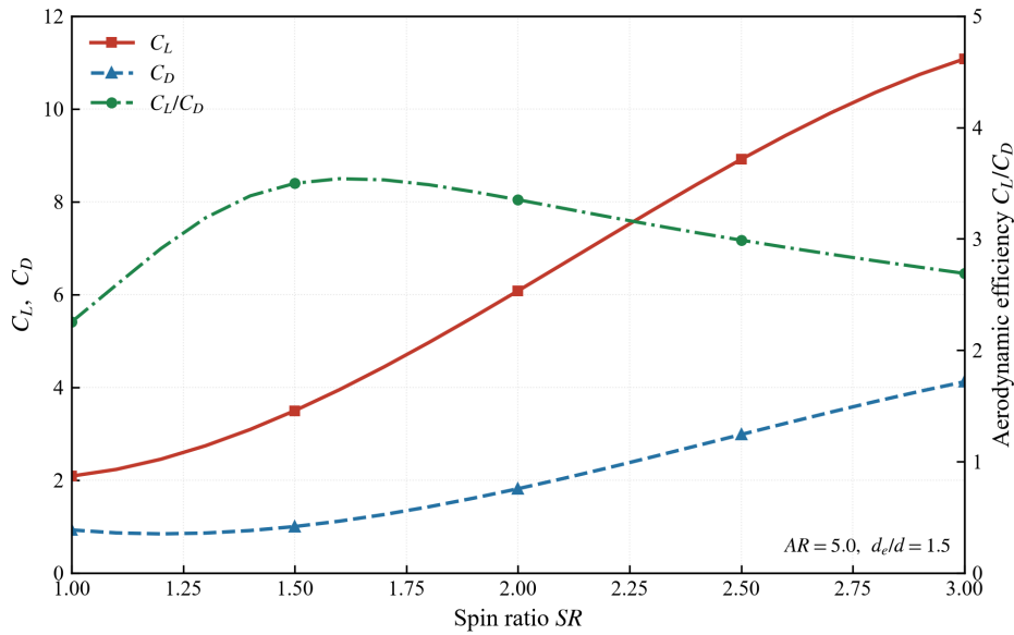
图 5 转筒帆升阻力系数与气动效率随转筒比的变化 ( AR = 5.0 , d_e/d = 1.5 )
