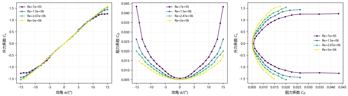
图 3 翼帆翼型极线的 XFOIL 计算结果
