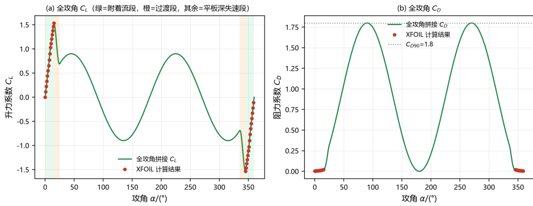
图 4 全攻角极线的三段式拼接结果
